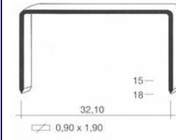
GRAPA 33 (SW-BOSS)
